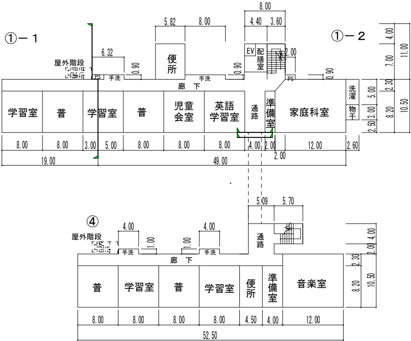
3階
