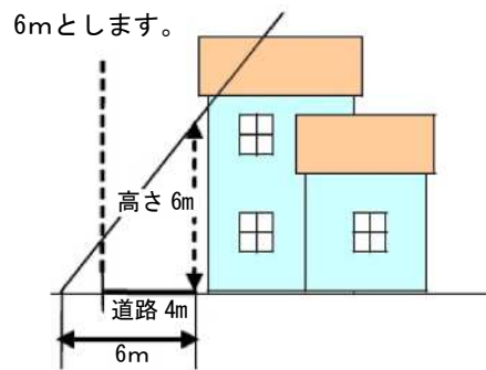
図 2-1 対象となる通行障害既存不適格建築物の高さ
