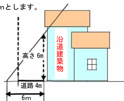
図 2-1 対象となる通行障害既存耐震不適格建築物の高さ
